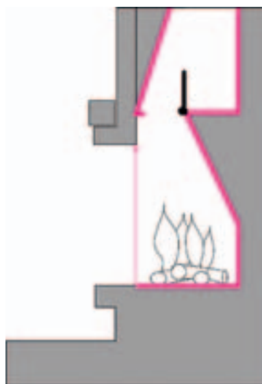
Obr. 1.5 Revoluční švédský vynález – kouřová křbová klapka
